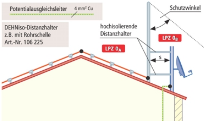
Bild 5: Antenne mit Fangstange und hochisolierenden Distanzhaltern auf Schrägdach bei Gebäuden mit Äußerem Blitzschutz
