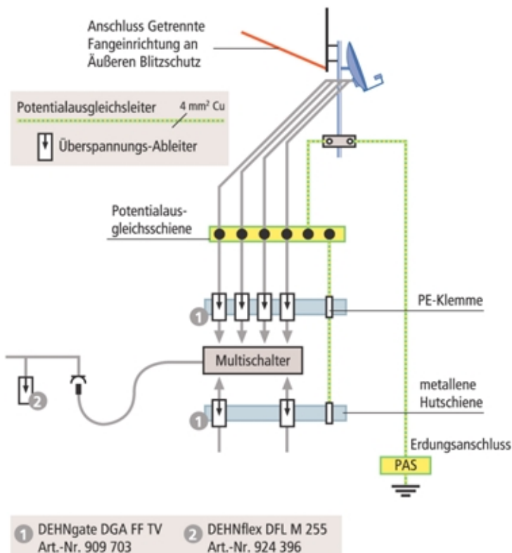
Bild 6: Überspannungs-Schutzgeräte nach der Potentialausgleichsschiene für die koaxialen Kabelschirme bei Antennenanlagen mit Äußerem Blitzschutz und Getrennter Fangeinrichtung
